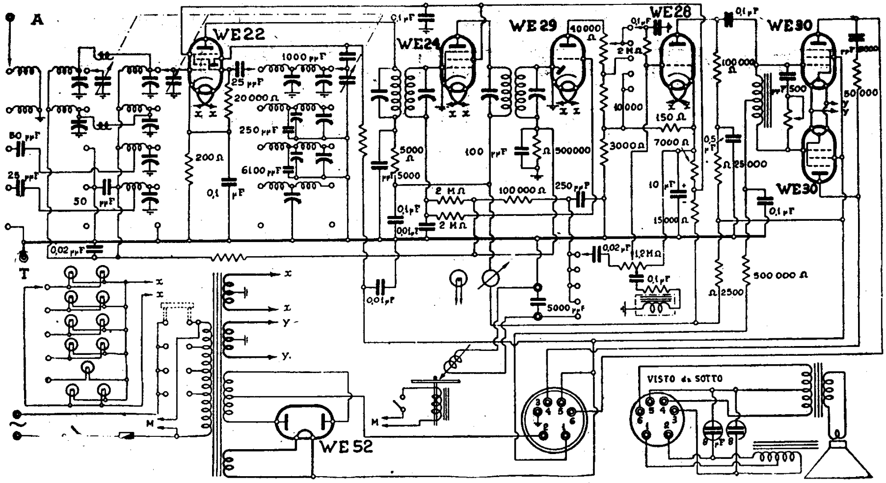
SIEMENS S. A. - MOD. « T 789 FONO »
